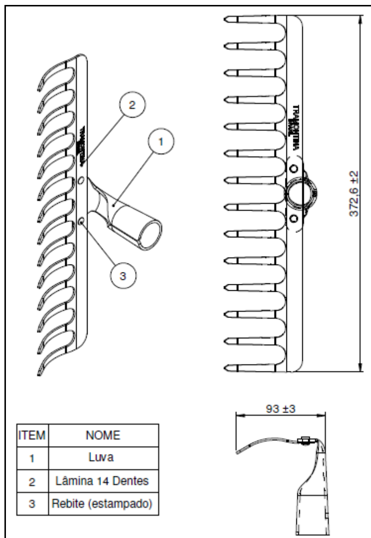
Figura 2 - Dimensional da lâmina del Rastrillo ref. 77101/144.
