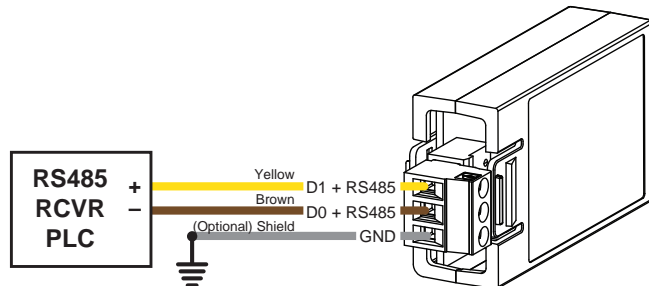
3-9950.395-M Modbus Module
