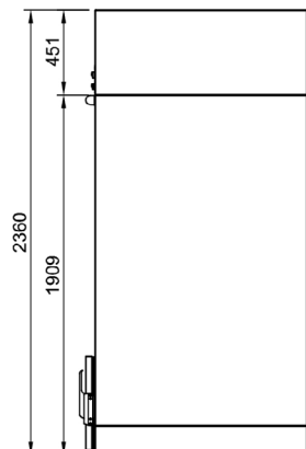
End Elevation
