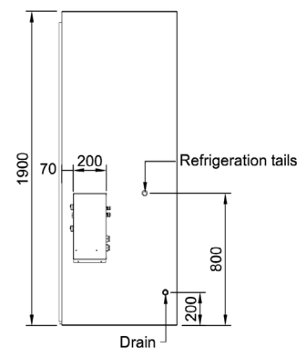
End Elevation
