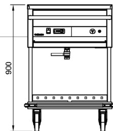
End Elevation
