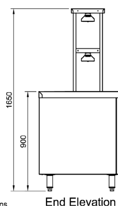
End Elevation
