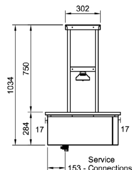
End Elevation
