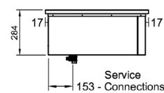
End Elevation
