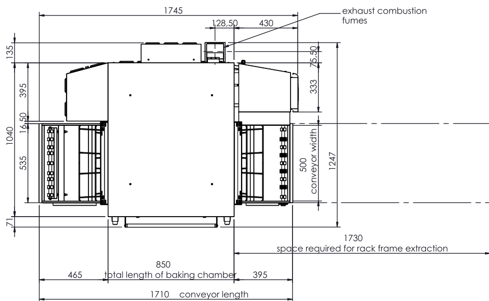
VISTA A SCALA 1 : 22
