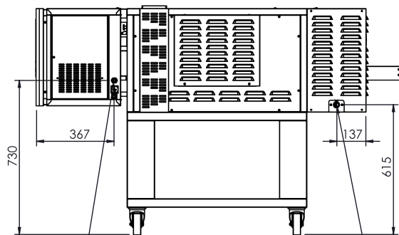
VISTA A SCALA 1 : 22
