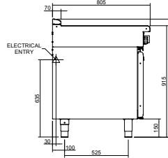
INLB8400R3 / INLB8400R5
