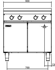
INLB8400R3 / INLB8400R5
