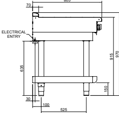
INLB8400R3 / INLB8400R5
