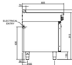
INLB8400R3 / INLB8400R5
