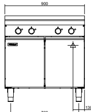
INLB8400R3 / INLB8400R5
