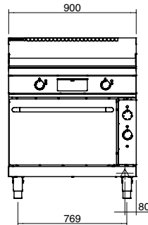
GP8910EC
