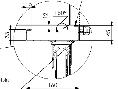
DETAIL AB SCALE 1 : 5
