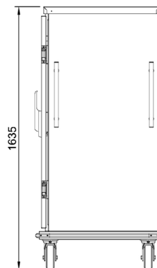
End Elevation
