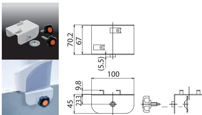
Partition Bracket NH-PST
