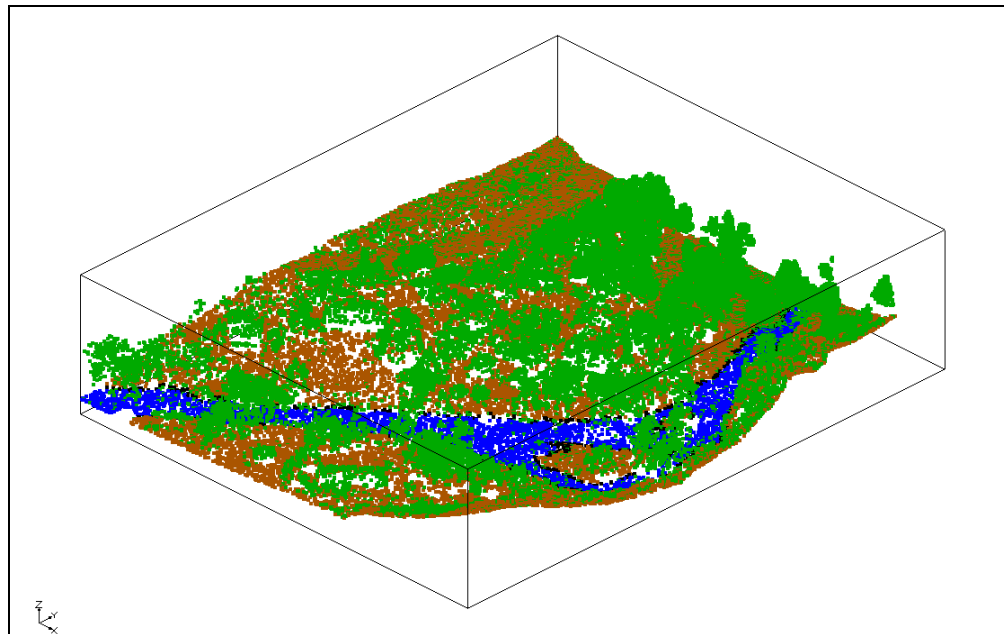
Figure 8 Trimmed lidar.
