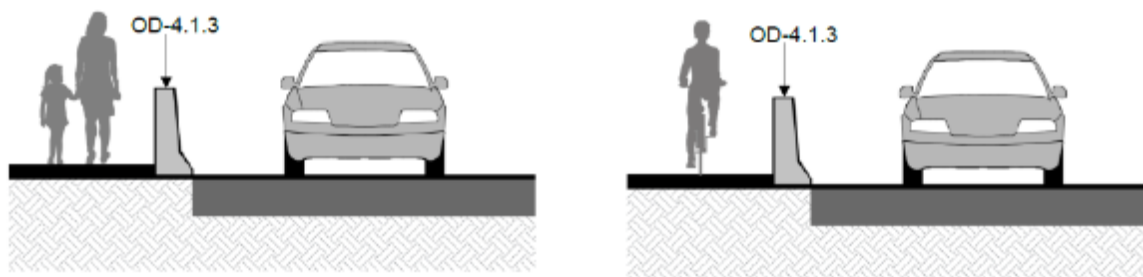
FIGURA 3.- Utilización de barreras de orilla de corona (OD-4.1) para proteger peatones y ciclistas
