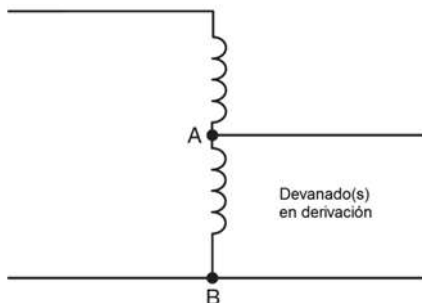
Figura 450-4.- Autotransformador
