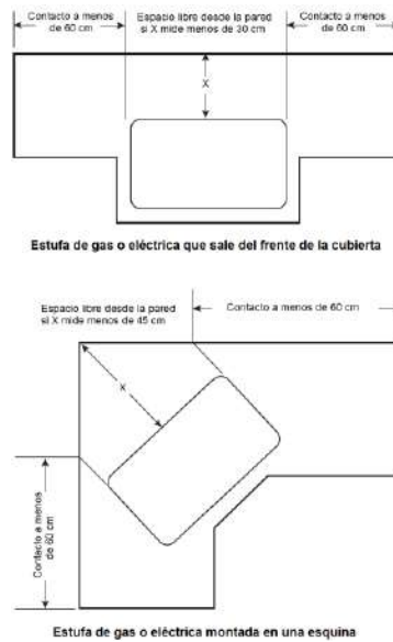
Figura 210-52(c)(1). - Determinación del área por detrás de una estufa, una parrilla montada en la cubierta o un fregadero
