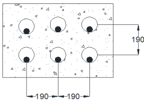
675 x 475 milímetros Banco de ductos eléctricos
