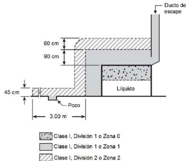
Figura 516-29(c).- Clasificación del área eléctrica para procesos abiertos de inmersión y recubrimiento, con ventilación y contención periférica parcial de vapores — Vapores NO confinados a equipos de procesos.
