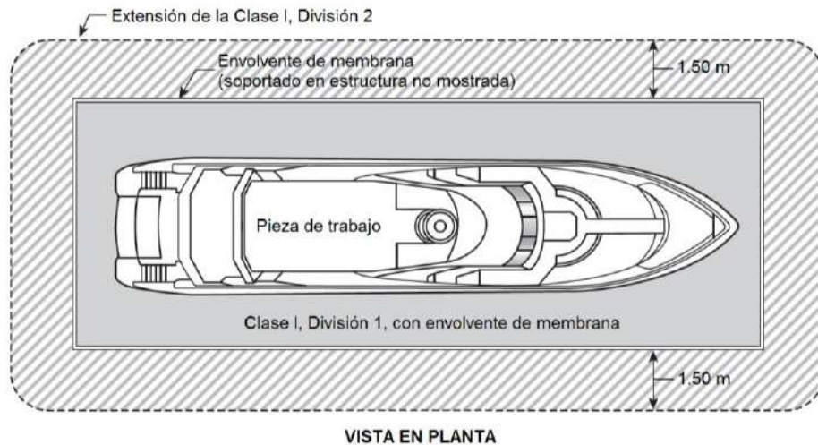
Figura 516-18.- Clasificación eléctrica para envoltorios exteriores temporales de membrana.
