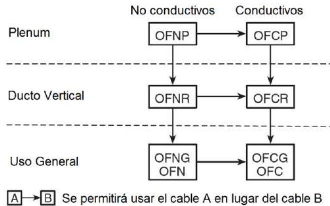
Figura 770-154.- Jerarquía de la sustitución de cables
