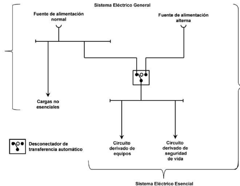
Figura 517-41(b).- Requisito mínimo un desconectador de transferencia para establecimientos de atención de enfermería y de atención limitada, para una demanda de hasta 150 kVA de los circuitos derivados de seguridad de vida y de equipos.
