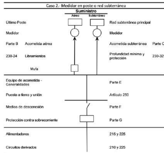
Figura 230-1.- Acometidas
