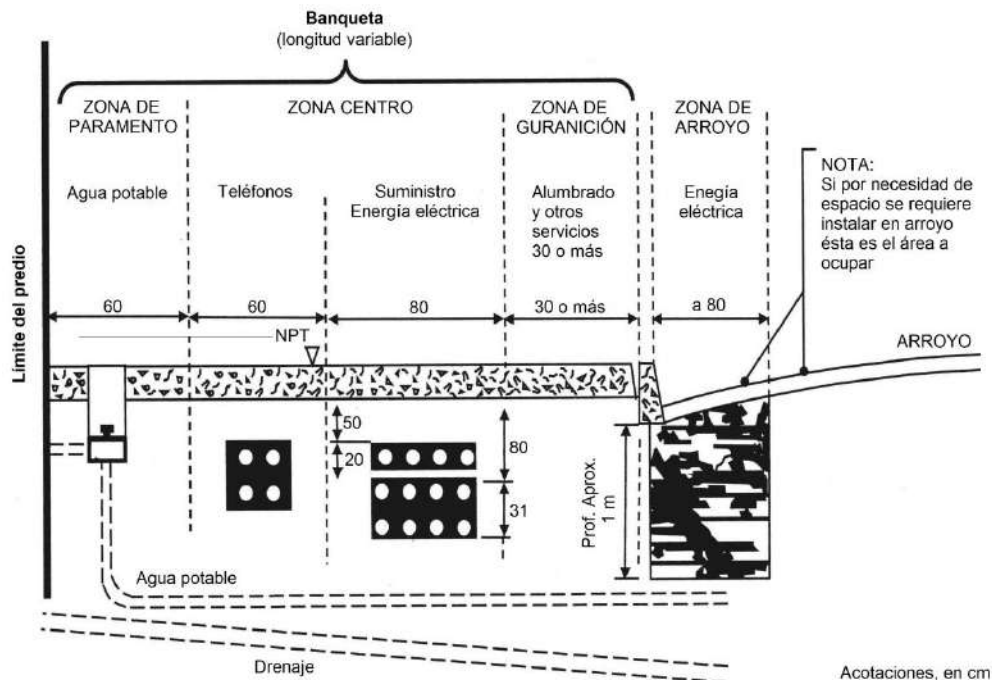
Figura 923-10(a)(3).- Zonificación recomendada de instalaciones en banqueta
