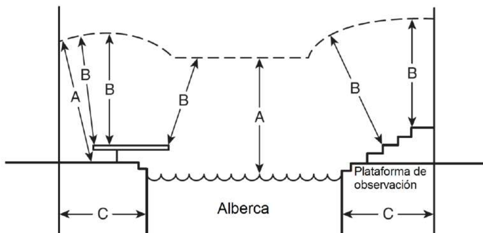
Figura 680-9(a).- Distancias desde las estructuras de la alberca
