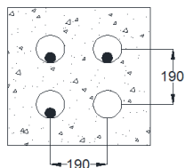
Detalle 2 475 x 475 milímetros Banco de ductos eléctricos Tres ductos eléctricos
