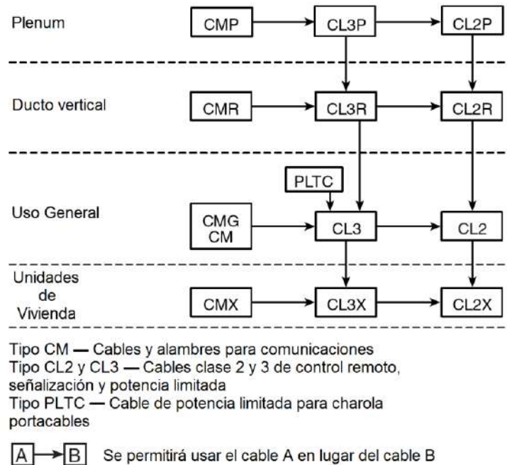
Figura 725-154(g).- Jerarquía de la sustitución de cables
