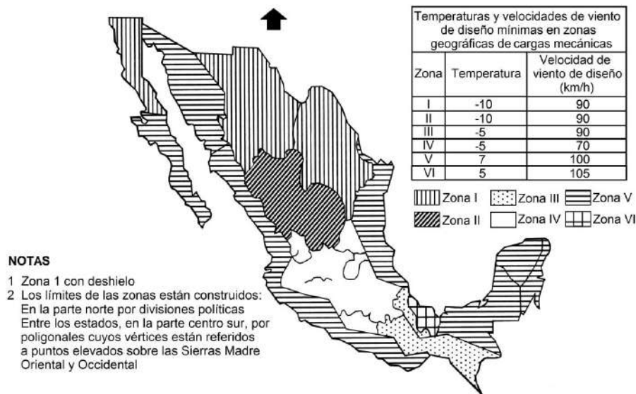
Figura 922-82.- Cálculo de cargas mecánicas
