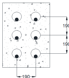
Detalle 3 475 x 675 milímetros Banco de ductos eléctricos Seis ductos eléctricos
