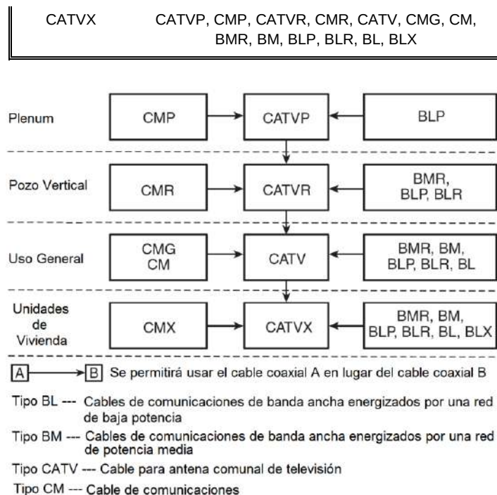
Figura 820-154.- Jerarquía de sustitución de cables
