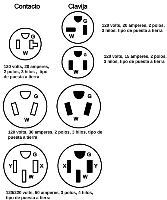
Figura 551-46(c)(1).- Configuraciones para contactos y clavijas de conexión del tipo puesta a tierra utilizadas con los cordones de alimentación de los vehículos de recreo y sus estacionamientos.
