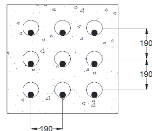
Detalle 4 675 x 675 milímetros Banco de ductos eléctricos Nueve ductos eléctricos
