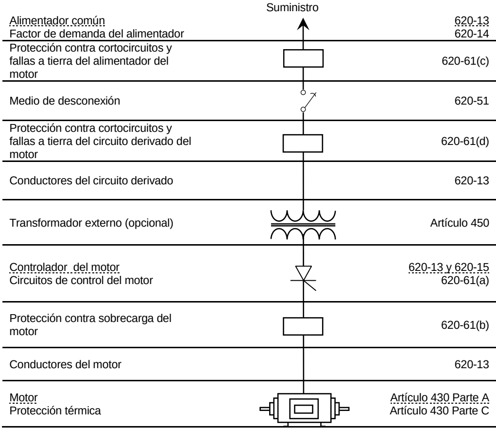
Figura 620-13.- Diagrama unifilar
