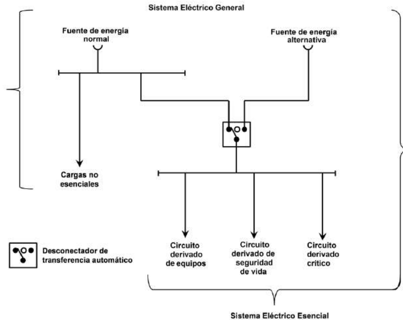
Figura 517-30 (b) requisitos mínimo de un desconectador de transferencia para hospitales y establecimientos para la atención médica de pacientes ambulatorios, con una demanda máxima de hasta 150 kVA de la carga conectada al sistema eléctrico esencial
