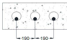
675 x 290 milímetros Banco de ductos eléctricos Tres ductos eléctricos
