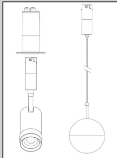
LINEAR CEILING / LINEAR PENDANT
