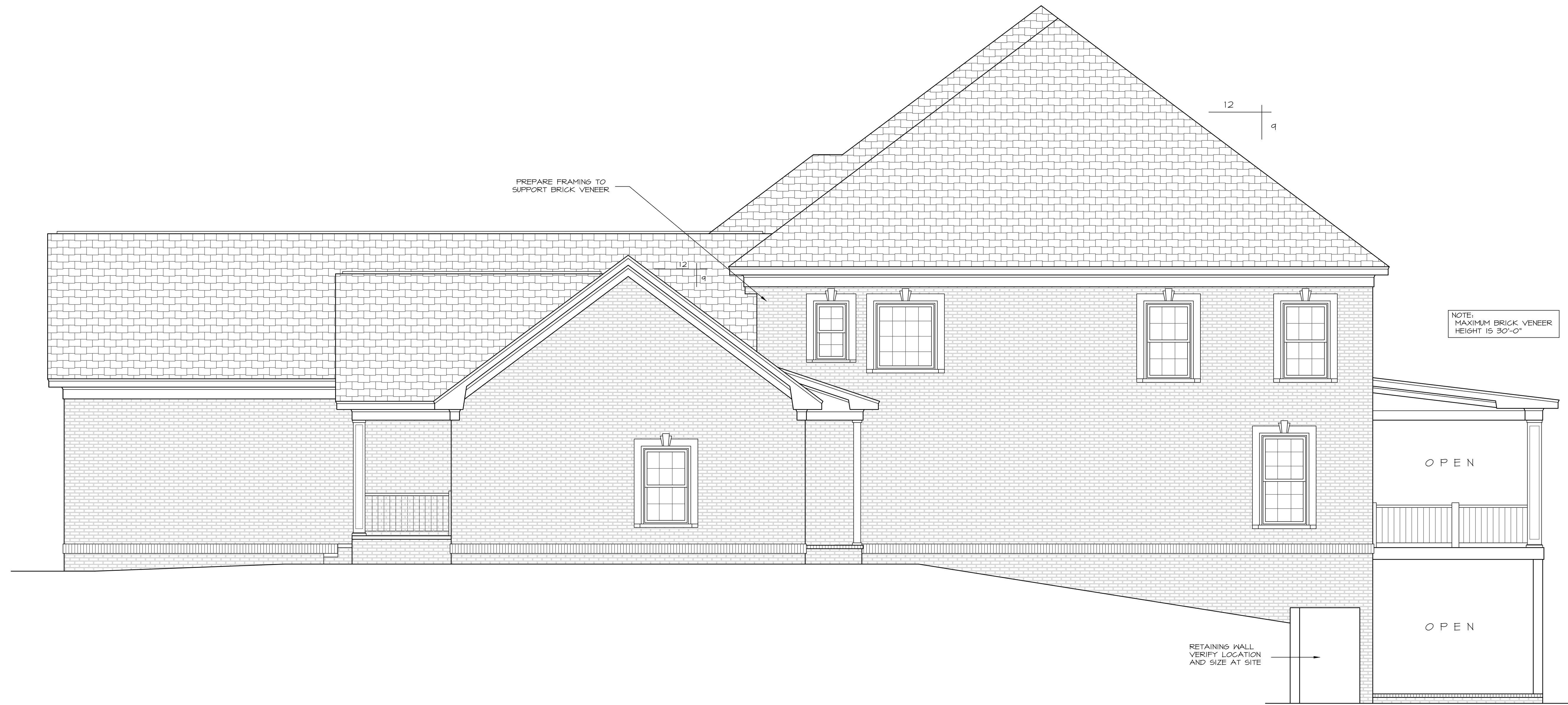
RIGHT ELEVATION
