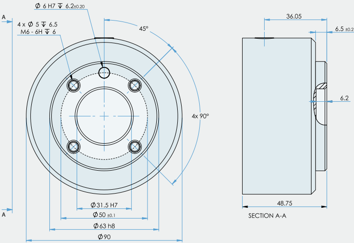
Tool flange for UR10e
