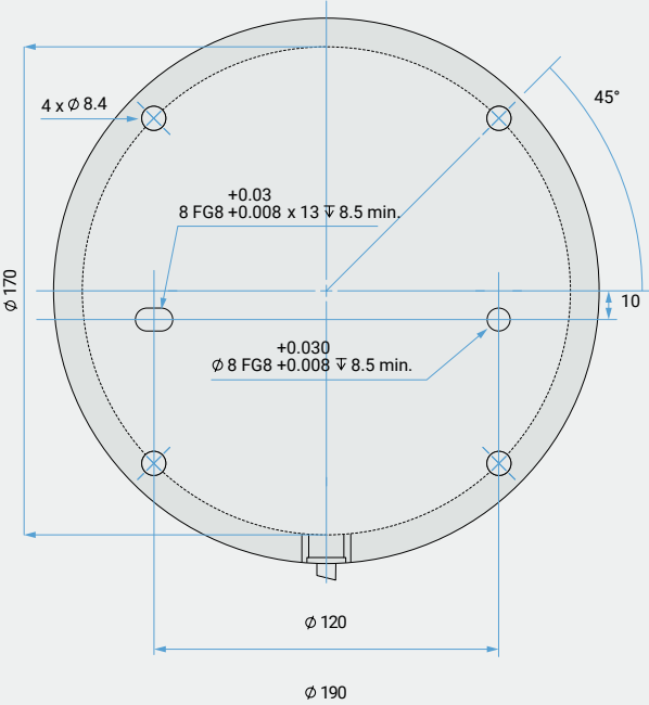
Tool flange for UR10e
