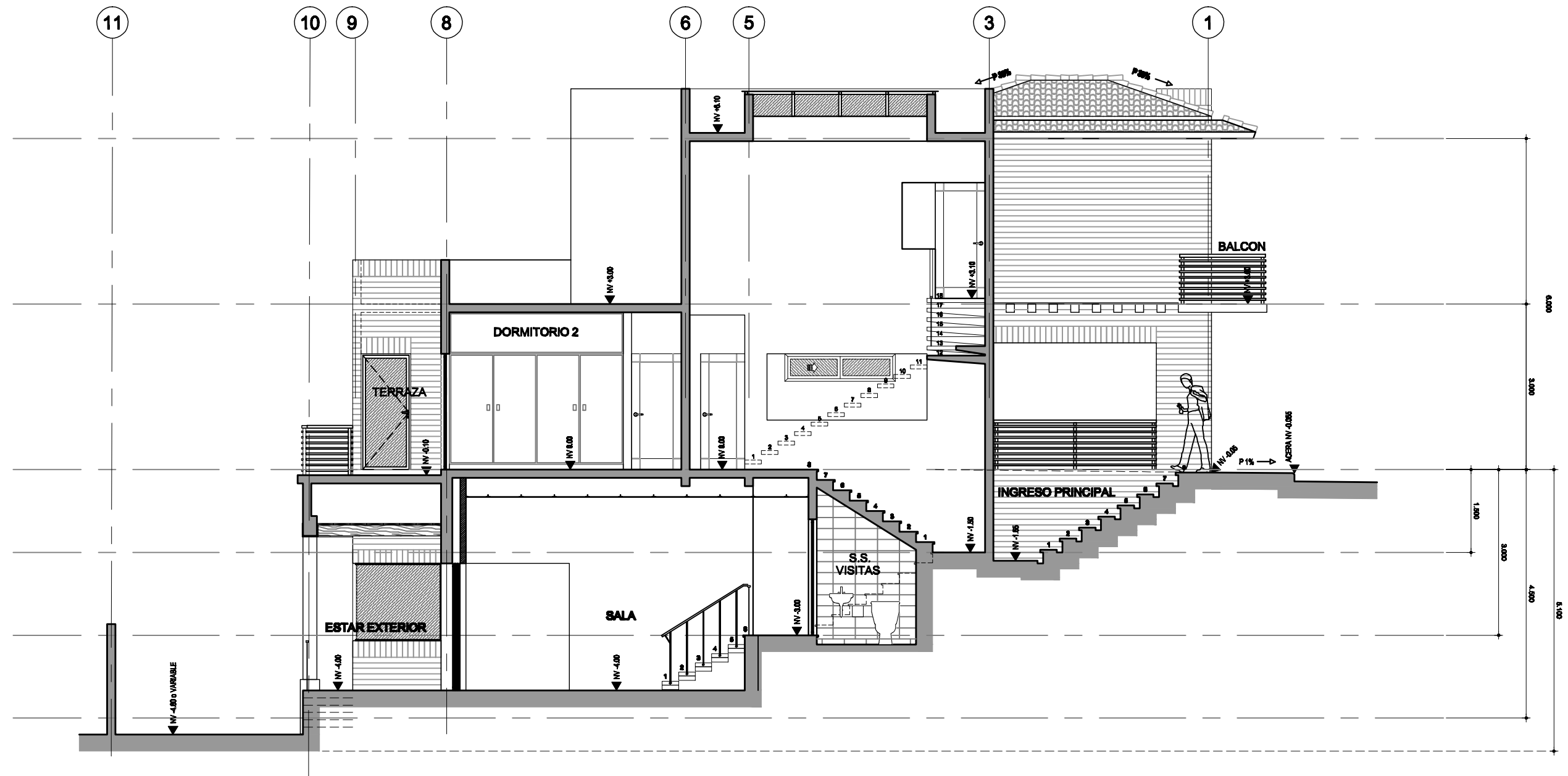
S1 SECCION 1: VISTA LONGITUDINAL ESCALA 1:125 CASA TIPO 03 IMPERIA
