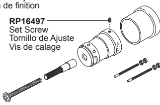
RP63686▲ Handle Assembly Ensamble de la Manija Poignée
