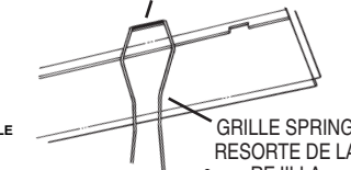
SLOT IN MOTOR PLATE RANURA EN EL PLACA DEL MOTOR
