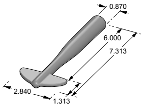
GK-6 – Gas key w/escutcheon.
