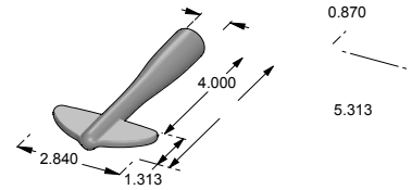
GK-4 – Gas key w/escutcheon.
