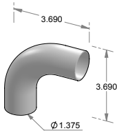
CLST-4E – Closet elbow.
