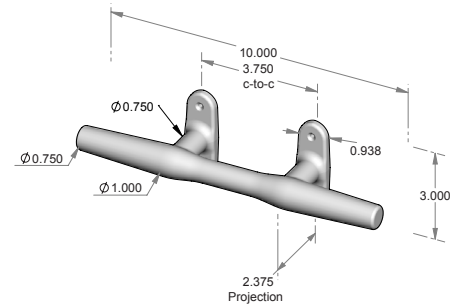
ANV-10 – Boat cleat.
