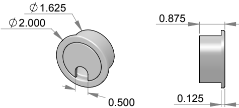
DKE-100 – Desk cord escutcheon.
