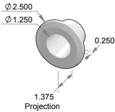
GK-ESC – Round gas key escutcheon.
