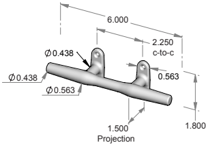
ANV-6 – Boat cleat.
