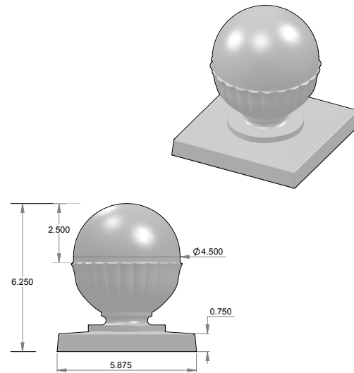
PF-101 – Post finial.
