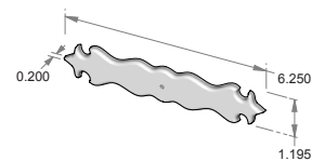
CKE-FDL – Fleur de Lis cabinet knob escutcheon. – 0.200" Thick.
