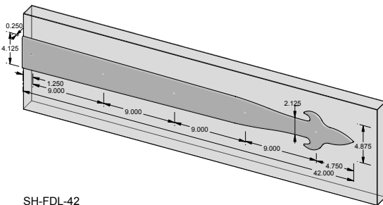
SH-FDL-42 – 42.000" Dummy Fleur de Lis strap hinge.
