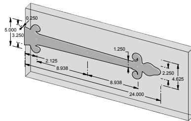
SH-FDL2-24 – 24.000" Dummy Fleur de Lis strap hinge.
