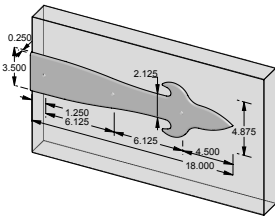
SH-FDL-18 – 18.000" Dummy Fleur de Lis strap hinge.
