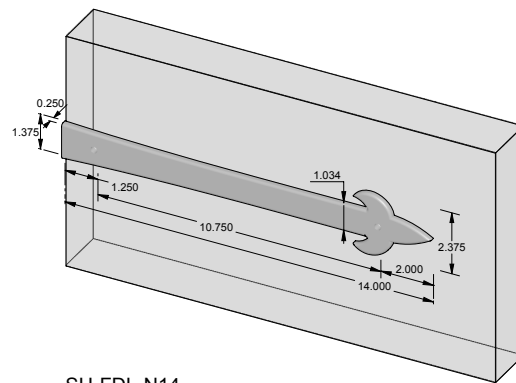
SH-FDL-N14 – 14.000" Dummy Narrow Fleur de Lis strap hinge.
