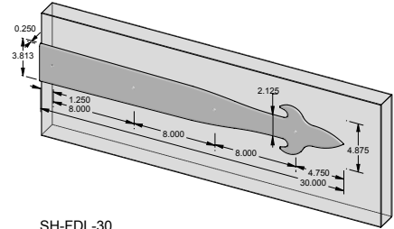
SH-FDL-30 – 30.000" Dummy Fleur de Lis strap hinge.
