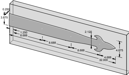
SH-FDL-32 – 32.000" Dummy Fleur de Lis strap hinge.
