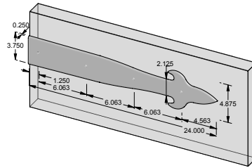
SH-FDL-24 – 24.000" Dummy Fleur de Lis strap hinge.
