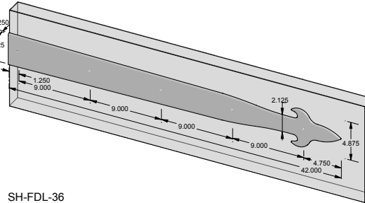
SH-FDL-36 – 36.000" Dummy Fleur de Lis strap hinge.
