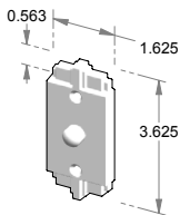
DRB-761 – Deco door bell plate. – Matching solid bronze button.
