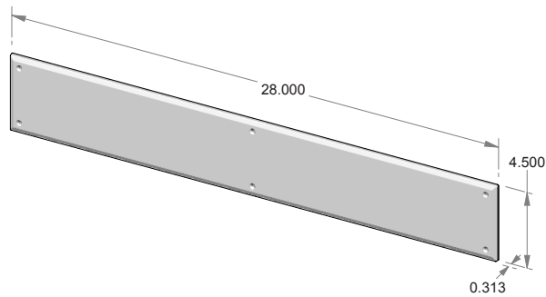
KP-284.5 – Bevel Edge kick plate.
