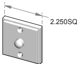
DRB-2101 – Mesa door bell plate. – Matching solid bronze button.
