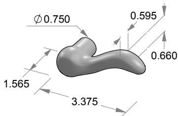
L-93 Chubster Lever
