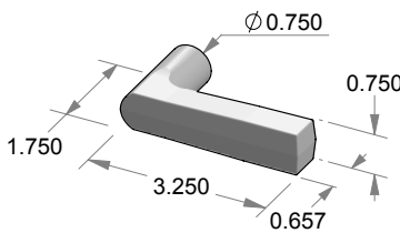
L-22 Mini Metro Lever
