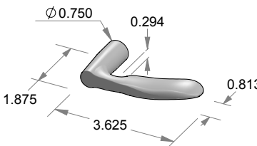
L-26 Mini Silver Creek Lever
