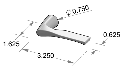
L-54 Mini Galena Lever
