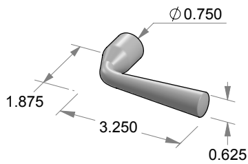
L-13/19 Mini Alturas/Muldoon Lever
