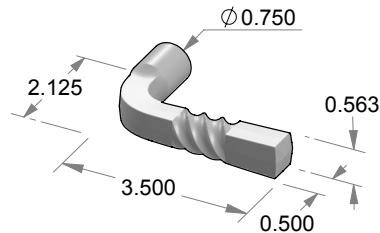
L-23 Mini Twist Lever
