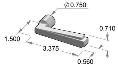
L-42 Mini Deco Lever
