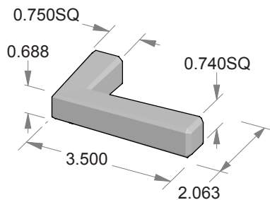
L-66SQ Mini Mesa Lever
