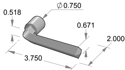
L-50 Mini Picabo Lever
