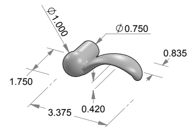
L-20 Mini Croy Lever
