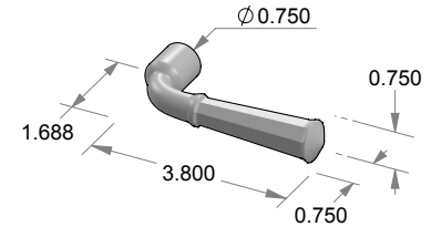
L-28 Mini Stanley Lever
