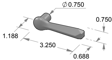
L-70 Mini Preston Lever
