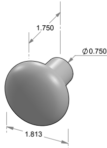
K-21 Mini Mushroom Knob
