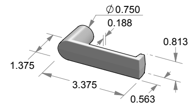
L-25 Mini Camas Lever
