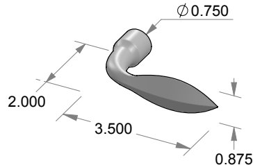
L-16 Mini Quigley Lever
