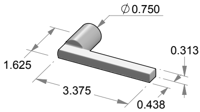
L-29 Mini Della Lever
