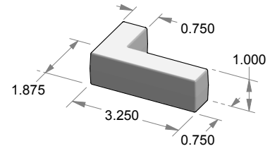
L-79SQ Mini Square Lever
