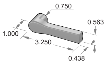
L-86 Tadpole Lever
