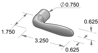
L-46 Mini Triumph Lever
