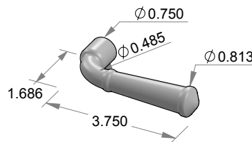
L-27 Mini Hailey Lever
