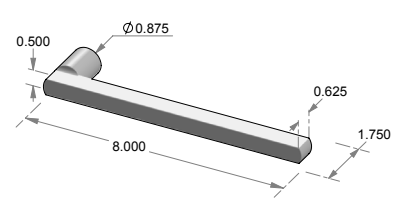
LS-129 Della lift & slide lever.
