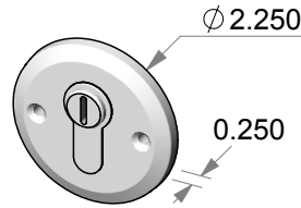
507ML-PROFILECYL Bevel Edge round cylinder trim.
