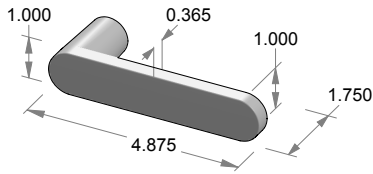
L-111 Flat Lever
