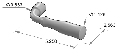
L-251 Cascade Lever
