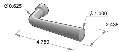
L-182-475 Titus Lever
