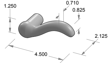
L-103 Chub Lever
