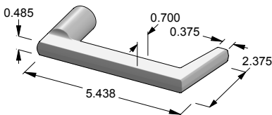
L-129OSR Della Lever w/Offset Return
