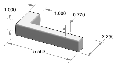
L-179SQ Ingot Lever* Square hub for use w/Novus escutcheon.
