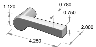
L-110 Baldy Lever
