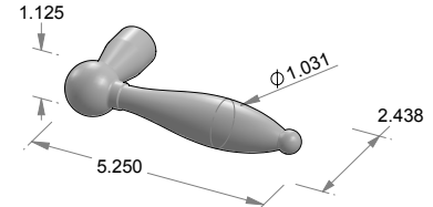
L-162 Hayden Lever
