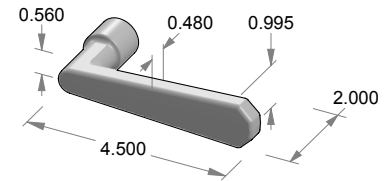
L-193 Pine Lever
