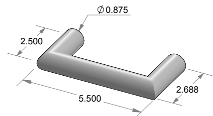
L-169R Lolo Lever w/Return
