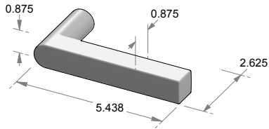
L-250 Lewis Lever
