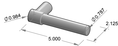
L-192 Potlatch Lever
