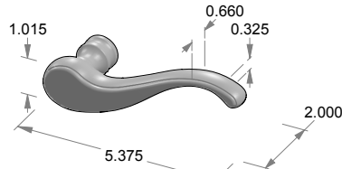
L-161 Lemhi Lever
