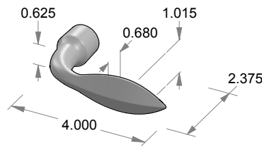
L-116 Quigley Lever t
