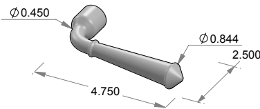
L-127 Hailey Lever
