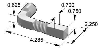
L-117 Twist Lever
