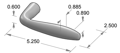
L-146 Triumph Lever
