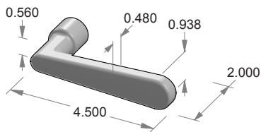
L-194 Pike Lever
