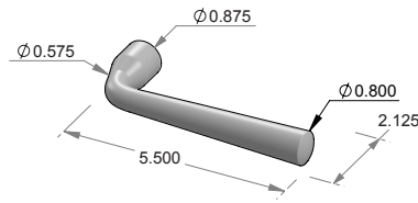
L-113-5.5 Alturas Lever
