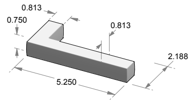
L-167SQ Elle Lever* Square hub for use w/Novus escutcheon.
