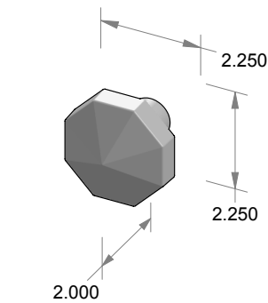
K-243 Latah Knob
