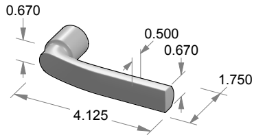
L-153 Alpen Lever
