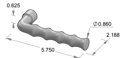
L-199 Orofino Lever
