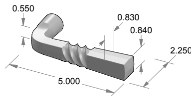
L-133 Revere Lever
