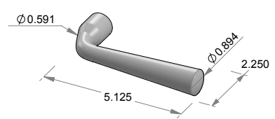
L-190 Easley Lever
