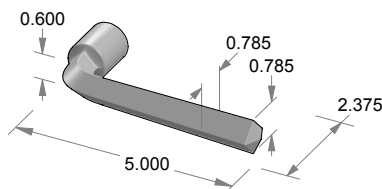
L-150 Picabo Lever
