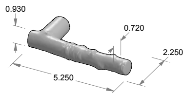
L-139 Aspen Lever
