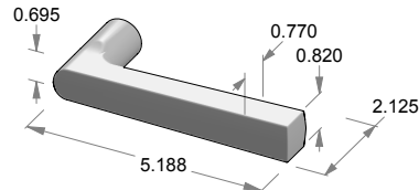
L-122 Metro Lever
