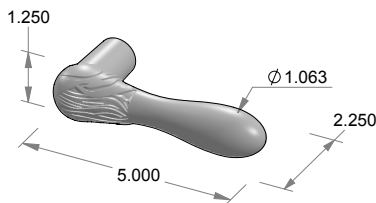
L-124 Carey Lever
