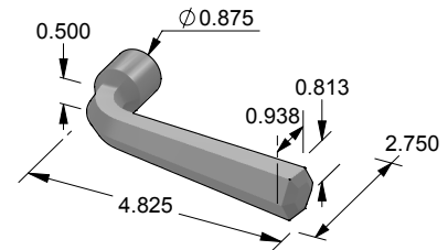
L-196 Gem Lever
