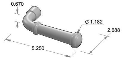
L-143 Harriman Lever
