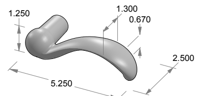
L-120 Croy Lever
