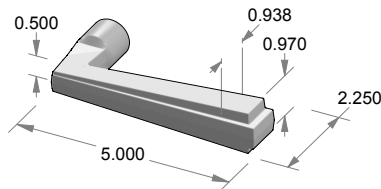
L-142 Deco Lever
