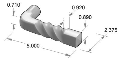
L-134 Mighty Twisted Lever
