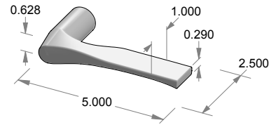
L-154 Galena Lever
