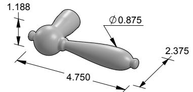
L-131 Tap Lever
