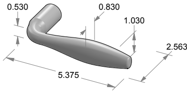
L-188 Keno Lever
