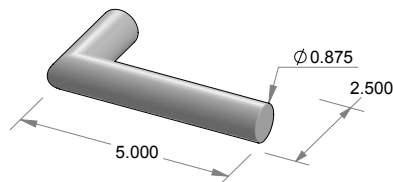
L-169 Lolo Lever
