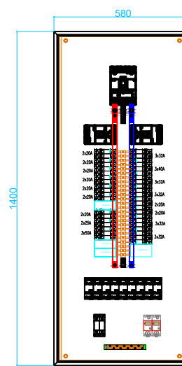
VISTA FRONTAL (SIN PUERTA / SIN MANDIL)
