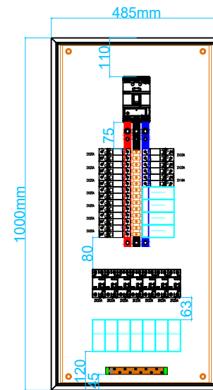
VISTA FRONTAL (SIN PUERTA / SIN MANDIL)
