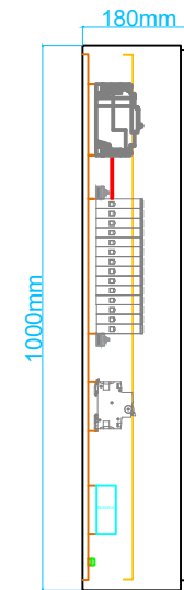
VISTA LATERAL
