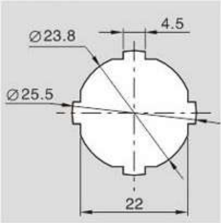
■ 开孔尺寸 Cut Out
