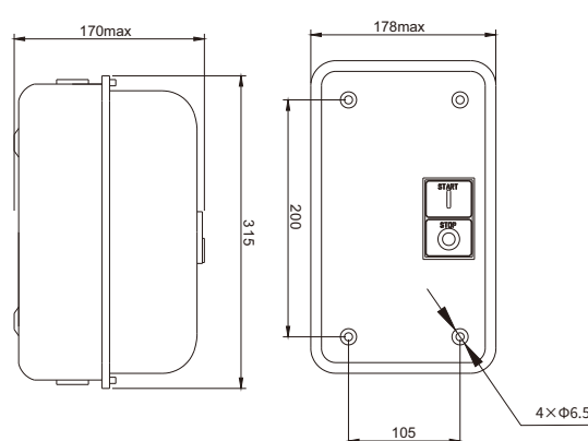
EKQ1-40~95(Steel base + Steel cover)
