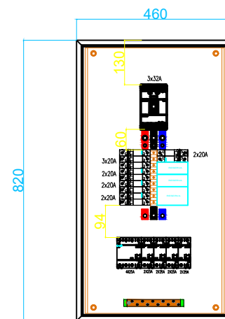
VISTA FRONTAL (SIN PUERTA / SIN MANDIL)
