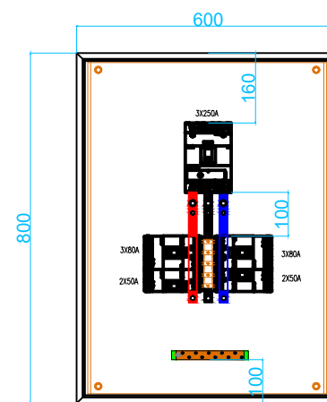
VISTA FRONTAL (SIN PUERTA / SIN MANDIL)
