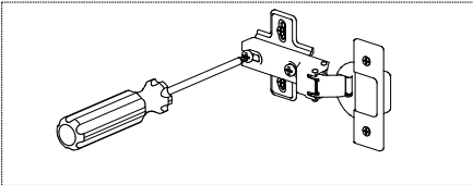
FAZER A JUNÇÃO DA DOBRADIÇA COM O CALÇO E APERTAR O PARAFUSO CENTRAL.
