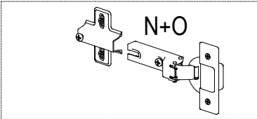
FIXAR A DOBRADIÇA NA PORTA COMO MOSTRA O DESENHO AO LADO.
