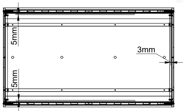
MEDIDAS DE MONTAGEM DO ESTRADO NA REGULAGEM INFERIOR.
