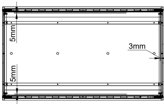
MEDIDAS DE MONTAGEM DO ESTRADO NA REGULAGEM INFERIOR.
