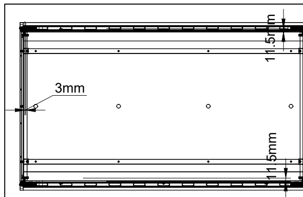
MEDIDAS DE MONTAGEM DO ESTRADO NA REGULAGEM SUPERIOR.
