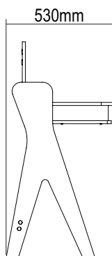
lateral/lado/side
