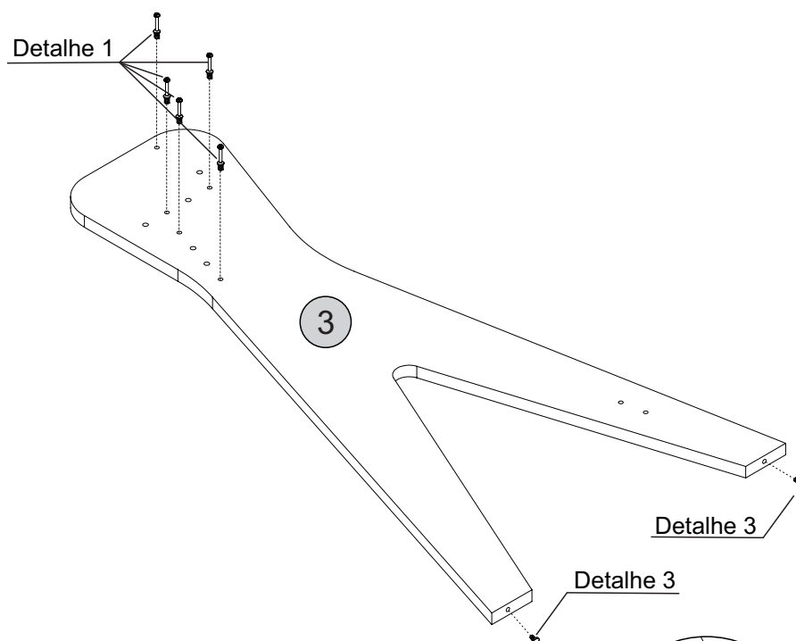
Detalhe 1 Detail/Detalle
