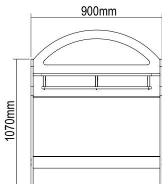
frente/frente/front
