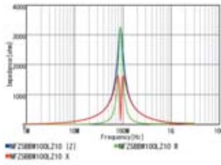
NFZ5BBW100LZ10
