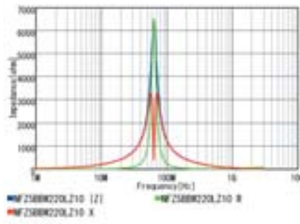
NFZ5BBW220LZ10
