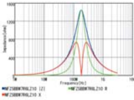
NFZ5BBW7R6LZ10
