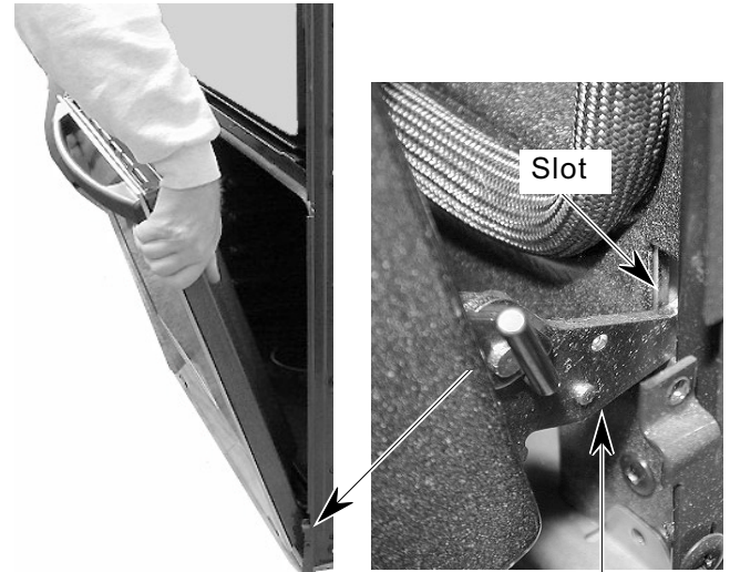
Hinge Hanger
