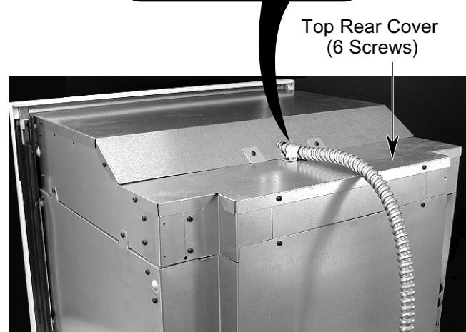
Conduit Clamp
