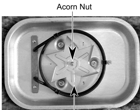
Convection Motor Fan
