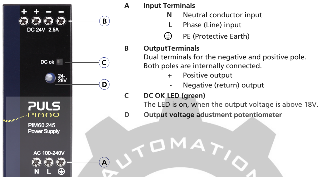
Fig. 13-1: Front side
