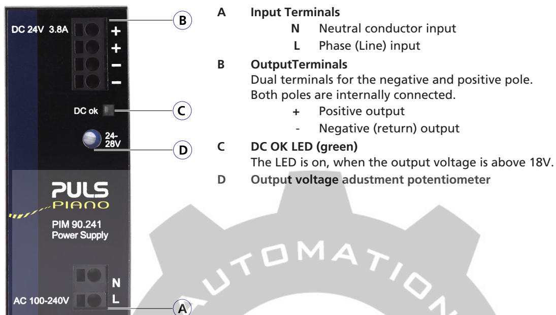
Fig. 13-1: Front side
