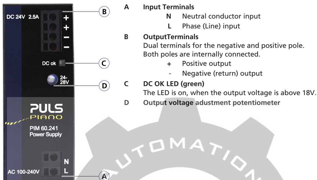
Fig. 13-1: Front side
