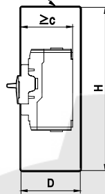
<Fig. 1> Clearances for Circuit Breaker / Espacio libre para el interruptor / Dégagements pour disjoncteur
