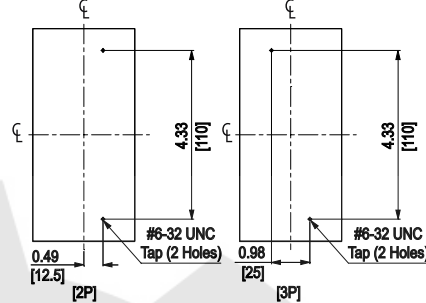
<Fig. 2> Circuit Breaker Mounting Bolt Drilling Plan / Plan de perforación de tornillo de montaje del interruptor / Plan de forage des Vis de montage du Disjoncteur
