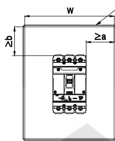
<Fig. 1> Clearances for Circuit Breaker / Espacio libre para el interruptor / Dégagements pour disjoncteur
