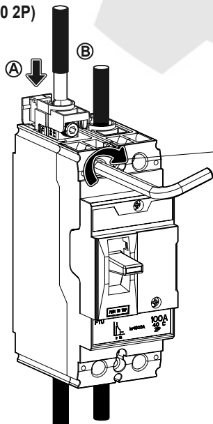
<Fig. 5> wire installation / instalación de cable / installation de fil.
