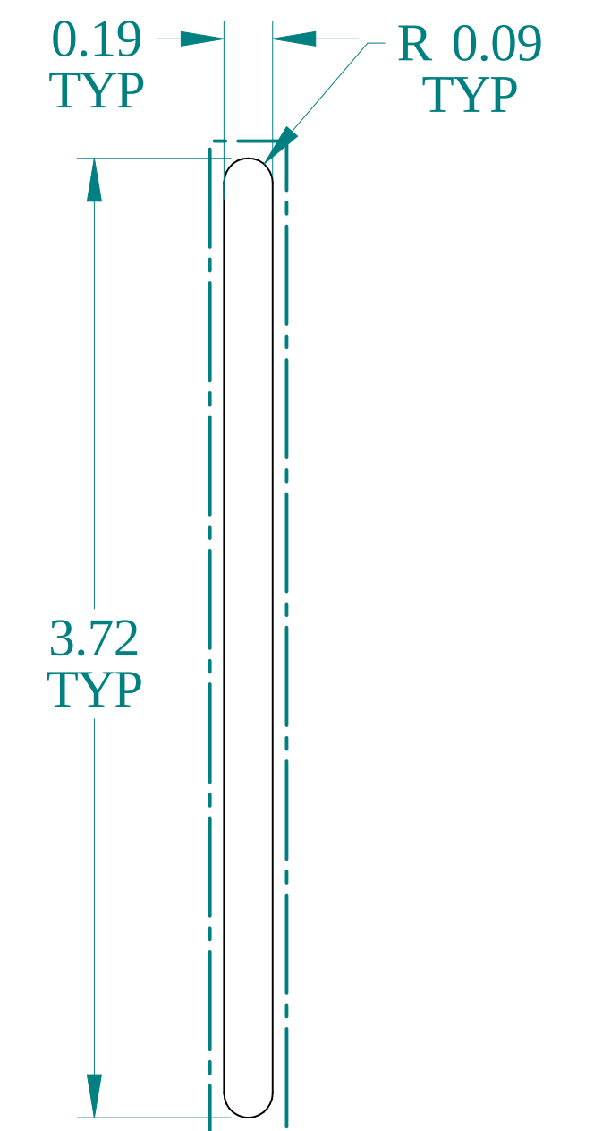
DETAIL Z TYP
